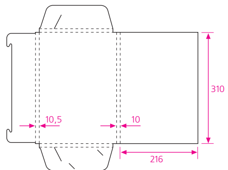
28 формат в развернутом виде 531,5 x 460 мм два замковых клапана
