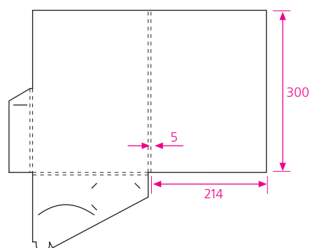
07 формат в развернутом виде 476,7 x 446,8 мм клапан замковый
