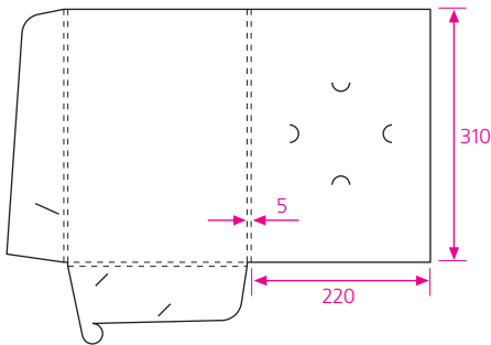
51 формат в развернутом виде 520 x 410 мм клапан замковый
