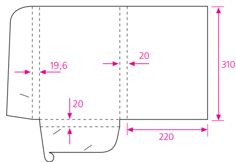
65 формат в развернутом виде 550 x 426 мм клапан замковый
