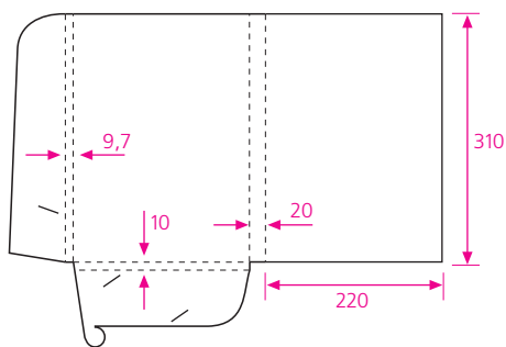
26 формат в развернутом виде 540 x 416 мм клапан замковый
