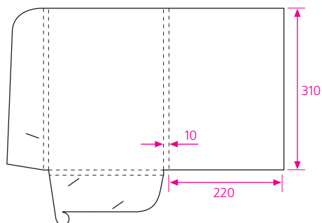
45 формат в развернутом виде 530 x 416 мм клапан замковый
