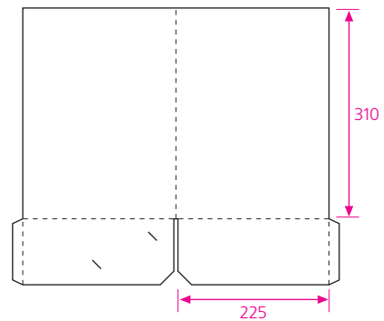
31 формат в развернутом виде 480 x 407 мм два клееных клапана
