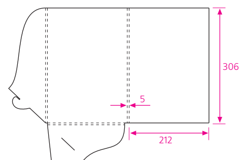
03 формат в развернутом виде 532 x 411 мм клапан замковый
