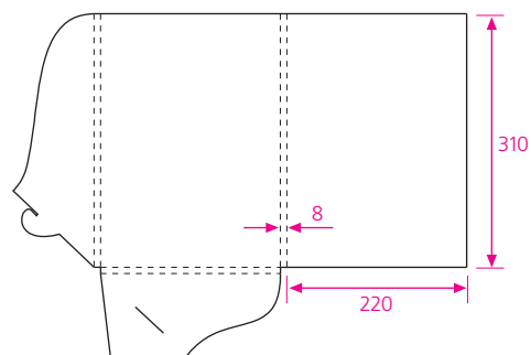
57 формат в развернутом виде 555 x 419 мм клапан замковый
