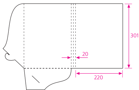
04 формат в развернутом виде 558 x 401 мм клапан замковый
