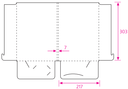
13 формат в развернутом виде 601 x 410 мм два замковых клапана
