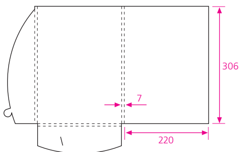
44 формат в развернутом виде 534 x 384 мм клапан замковый
