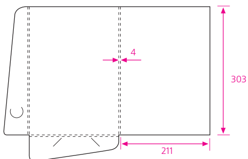
69 формат в развернутом виде 486 x 365 мм клапан замковый
