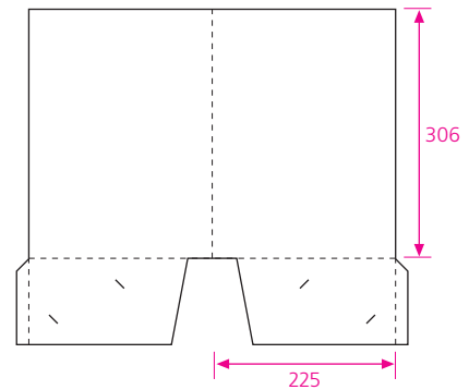
17 формат в развернутом виде 480 x 412 мм два клееных клапана
