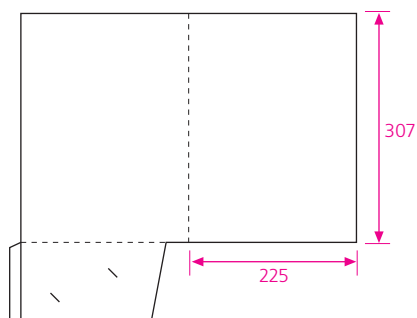
10 формат в развернутом виде 465 x 412 мм клапан клееный
