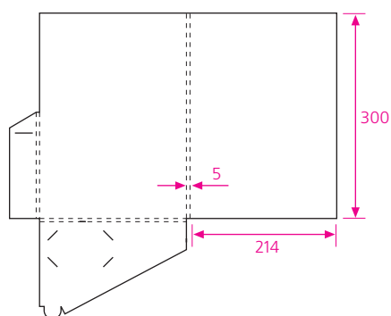
06 формат в развернутом виде 476,7 x 446,8 мм клапан замковый
