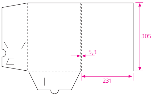
66 формат в развернутом виде 586,3 x 407,5 мм клапан замковый
