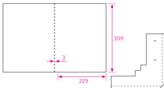
41 формат в развернутом виде 585 x 407 мм клапан клееный (вырубается отдельно)
