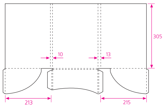
27 формат в развернутом виде 685 x 425 мм
