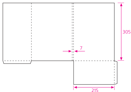
35 формат в развернутом виде 601 x 430 мм два клееных клапана
