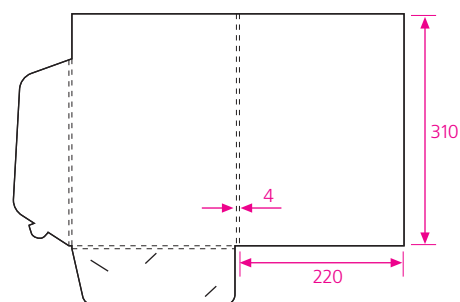
18 формат в развернутом виде 522 x 389 мм клапан замковый
