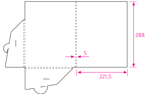
32 формат в развернутом виде 541,4 x 405 мм клапан замковый
