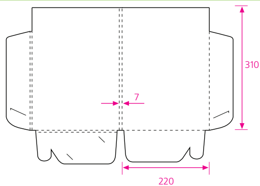
71 формат в развернутом виде 572 x 395 мм два замковых клапана
